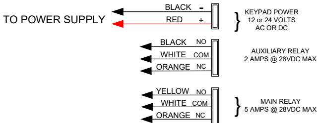
Fig. 2 Wiring Pigtail Color Code
